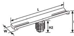
TapeClip TC2FT6LG
